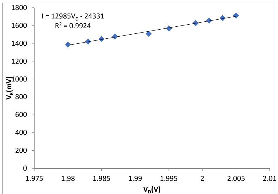
ภาพ 7 กราฟแสดงศักย์เริ่มต้น LED สีเขียว โดยใช้ 10 ค่าสุดท้าย จากสมการ I = 12985V_D - 24331 เมื่อ I=0 จะได้ V_D=1.874 V
