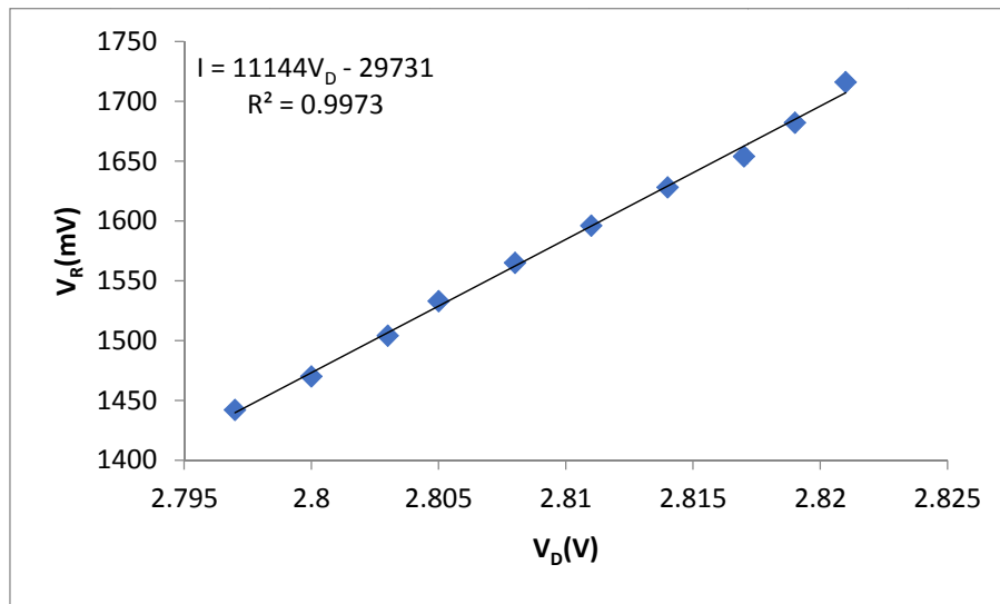
ภาพ 8 กราฟแสดงศักย์เริ่มต้นLED สีฟ้า โดยใช้ 10 ค่าสุดท้าย จากสมการ I = 11144V_D - 29731 เมื่อ I=0 จะได้ V_D=2.668 V
