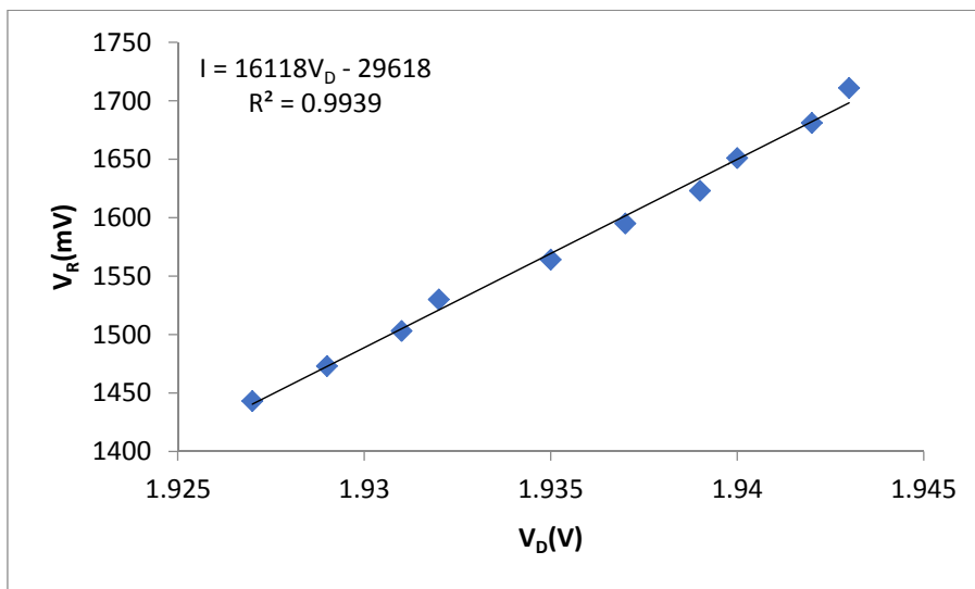
ภาพ 5 กราฟแสดงศักย์เริ่มต้นLED สีแดง โดยใช้ 10 ค่าสุดท้าย จากสมการ I = 16118V_D - 29618 เมื่อ I=0 จะได้ V_D=1.838 V
