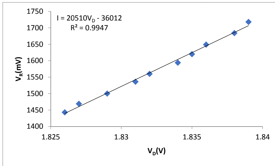
ภาพ 6 กราฟแสดงศักย์เริ่มต้น LED สีส้ม โดยใช้ 10 ค่าสุดท้าย จากสมการ I = 20510V_D - 36012 เมื่อ I=0 จะได้ V_D=1.756 V
