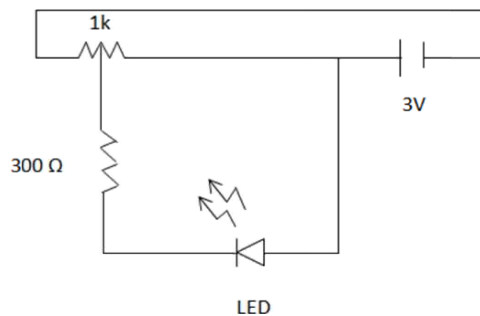
ภาพ 2 วงจรการทดลองวัดค่าคงที่ของแพลงค์ด้วย LED
