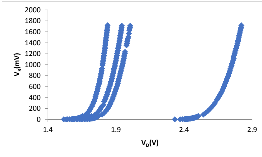
ภาพ 4 กราฟแสดงผลค่า VR และ VD ทั้ง 4 สี
