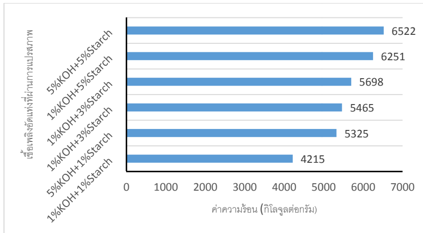
ภาพ 3 ค่าความร้อนของเชื้อเพลิงอัดแท่งที่ผ่านการคาร์บอนไนเซชันที่สภาวะต่างๆ
