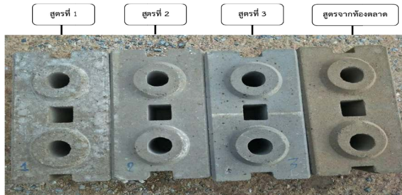
ภาพ 4 อิฐบล็อกประสานที่มีส่วนผสมของเถ้ากะลามะพร้าวแต่ละสูตรกับอิฐบล็อกจากท้องถิ่น
