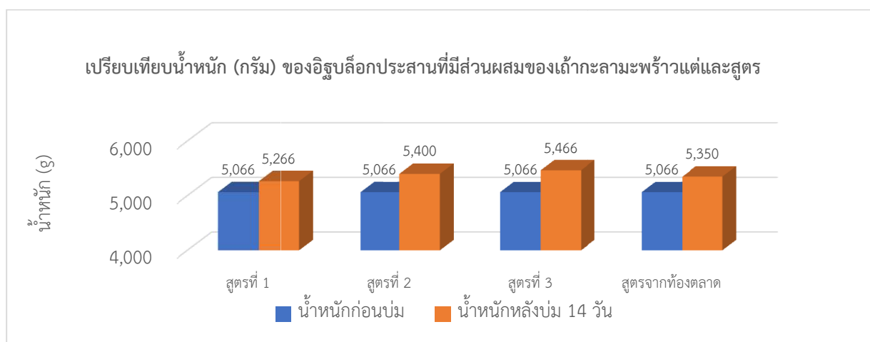
ภาพ 6 แสดงการเปรียบเทียบน้ำหนัก (กรัม) ของอิฐบล็อกประสานที่มีส่วนผสมของเถ้ากละมะพร้าวแต่ละสูตร
