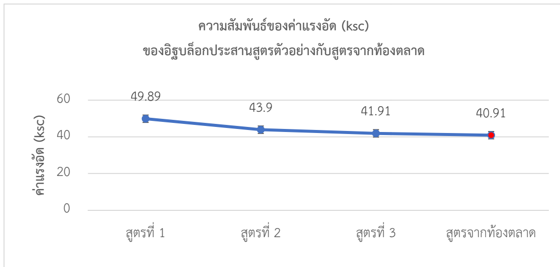
ภาพ 7 แสดงความสัมพันธของค่าแรงอัด (ksc) ของอิฐบล็อกประสานสูตรตัวอย่างกับสูตรจากท้องตลาด
