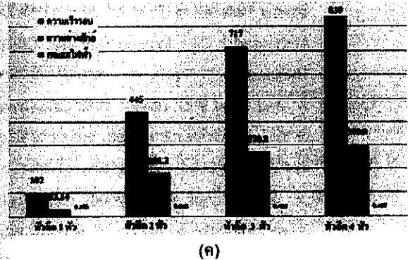
ภาพที่ 5 ความเร็วรอบ (rpm) ความต่างศักย์ไฟฟ้า (V) และกระแสไฟฟ้า (mA) ที่ได้จากการทดสอบชุดกังหันน้ำผลิตไฟฟ้าขนาดจิ๋วแบบหัวฉีดอย่างง่ายจากมอเตอร์เครื่องซักผ้า (ก) จำนวนใบพัด 12 ใบ (ข) จำนวนใบพัด 15 ใบ และ (ค) จำนวนใบพัด 18 ใบ
