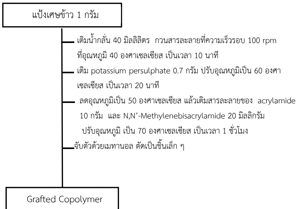
แผนผังที่ 1 แสดงขั้นตอนการเตรียมพอลิเมอร์ไฮโดรเจล (Adair, 2017)
