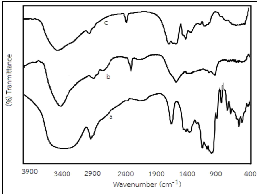
แผนภาพ 1 แสดงสเปกตรัมของ FTIR (a) แปะจากเศษข้าว (b) กราฟต์โคพอลิเมอร์ของแปะจากเศษข้าวและพอลิอะคริลาไมด์ และ (c) กราฟต์โคพอลิเมอร์ของแปะจากเศษข้าวและพอลิอะคริลาไมด์หลังจากทำปฏิกิริยากับ 2M NaOH และล้างด้วยน้ำกลั่น
