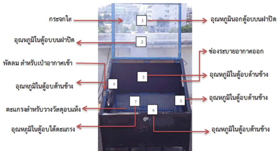
ภาพ 1 ลักษณะห้องลดความชื้นและตำแหน่งวัดอุณหภูมิของเครื่องลดความชื้นขึ้นส้มแขกพลังงานแสงอาทิตย์อย่างง่าย
