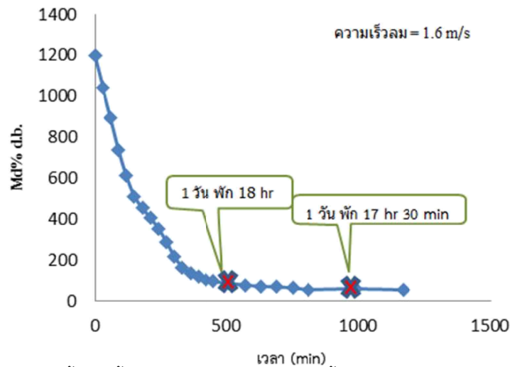
ภาพ 5 การเปลี่ยนแปลงความชื้นของชิ้นสัมแชกระหว่างการลดความชื้นด้วยเครื่องอบแห้งพลังงานแสงอาทิตย์อย่างง่าย
