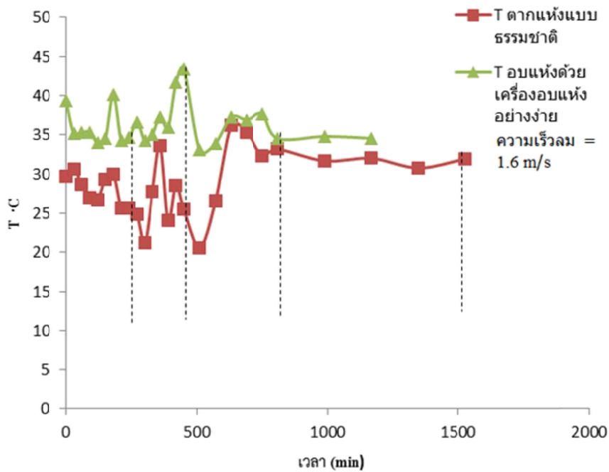
ภาพ 6 การเปลี่ยนแปลงอุณหภูมิที่ผิวของชิ้นส้มแซกระหว่างการลดความชื้นโดยการตากแห้งแบบธรรมชาติและการลดความชื้นด้วยเครื่องลดความชื้นพลังงานแสงอาทิตย์อย่างง่าย
