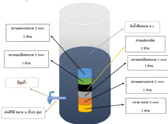
ภาพ 2 ชุดเครื่องกรองน้ำประติษฐ์โดยวิธีการกรองแบบไส้กรอง
