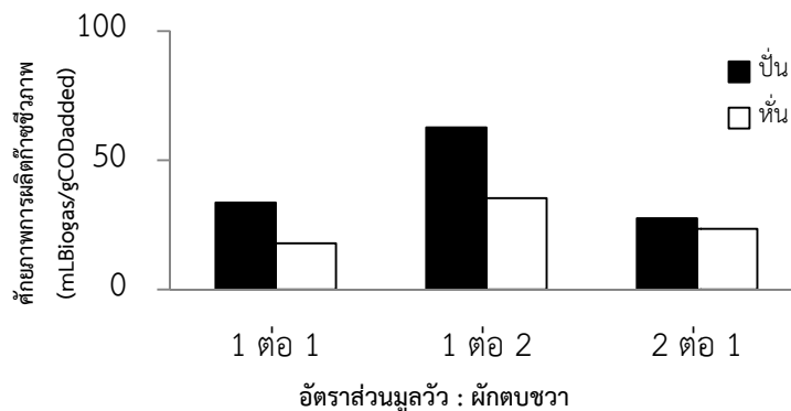
ภาพ 7 ศักยภาพในการผลิตก๊าซชีวภาพ
