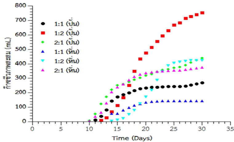
ภาพ 6 ปริมาณก๊าซชีวภาพสะสม
