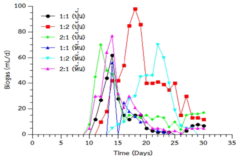
ภาพ 5 อัตราการเกิดก๊าซชีวภาพ
