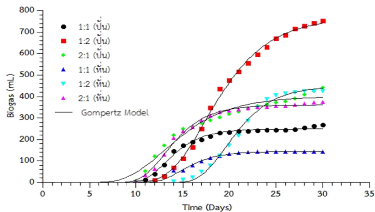
ภาพ 8 การเปรียบเทียบผลการทดลองกับ modified Gompertz model
