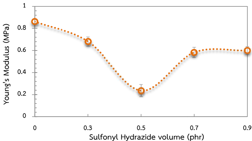
ภาพ 4 ความสัมพันธ์ระหว่างค่า Young's Modulus กับปริมาณสาร Sulfonfyl Hydrazide
