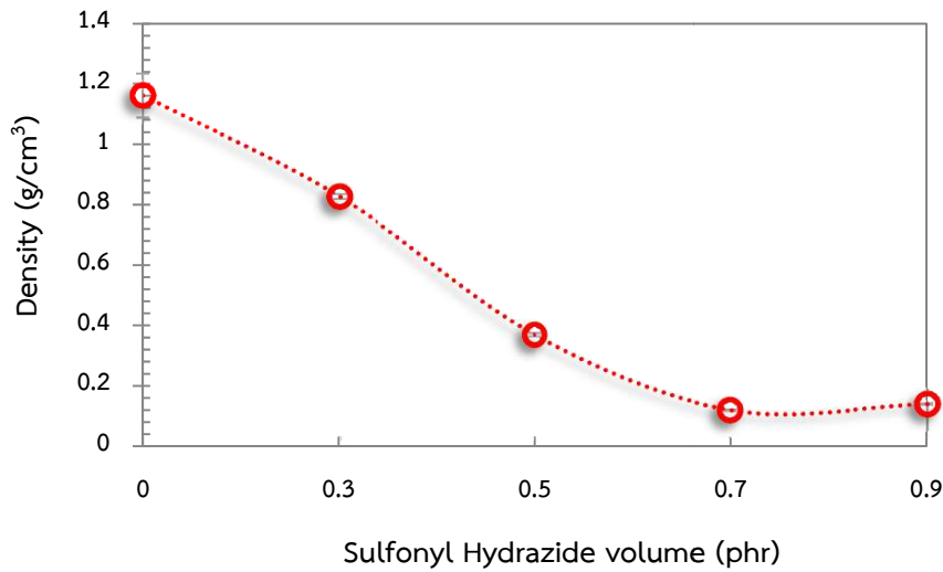
ภาพ 3 ความสัมพันธ์ระหว่างความหนาแน่นกับปริมาณสาร Sulfonfyl Hydrazide
