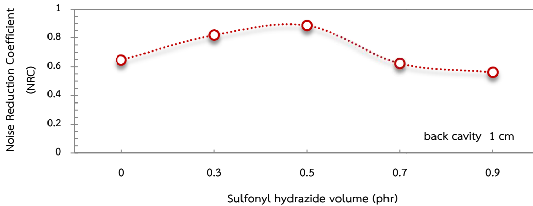
ภาพ 7 ค่าการลดระดับเสียงของโฟมยางธรรมชาติในแต่ละสัดส่วนการผสม
