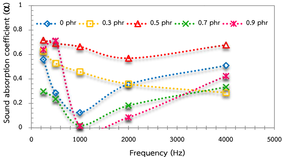
ภาพ 5 ความสัมพันธ์ระหว่างสัมประสิทธิ์การดูดซับเสียงที่ความถี่ต่างๆ
