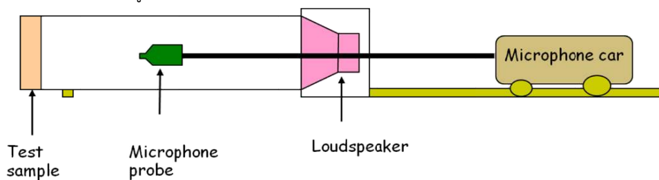
ภาพ 1 ชุดทดสอบสมบัติการดูดซับเสียงด้วยเทคนิคท่อคลื่นนิ่ง
