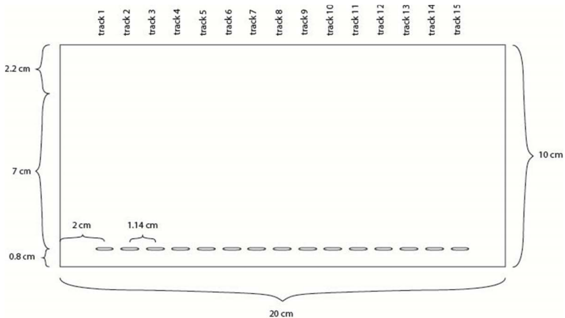
ภาพ 1 รูปแบบการฉีดพ่นสารบนแผ่น TLC สมรรถนะสูง
