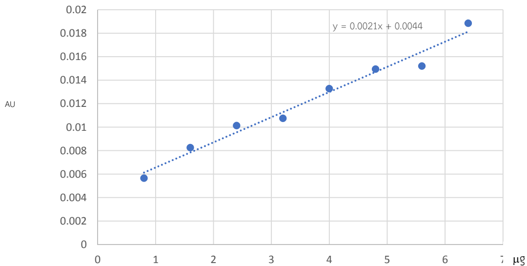
ภาพ 8 กราฟมาตรฐานเคอร์ซีติน
