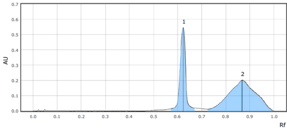
ภาพ 5 โครมาโทแกรมของสารมาตรฐานเคอร์ชิติน
